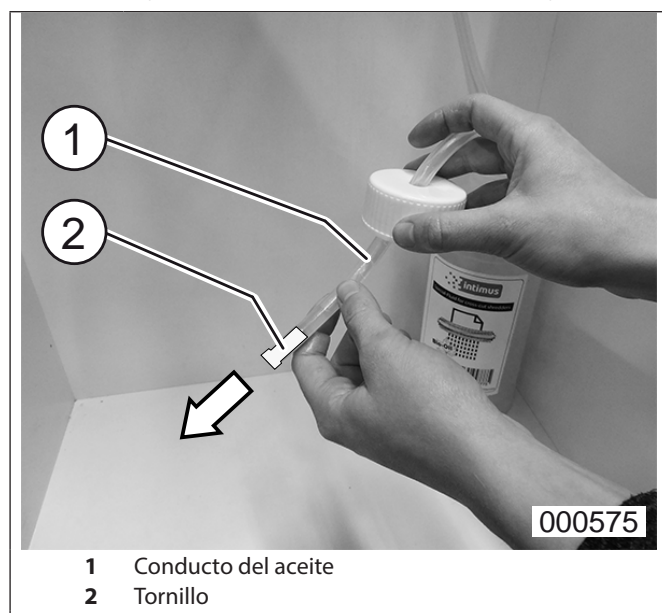
Fig. 1 Instalación del sistema de lubricación
