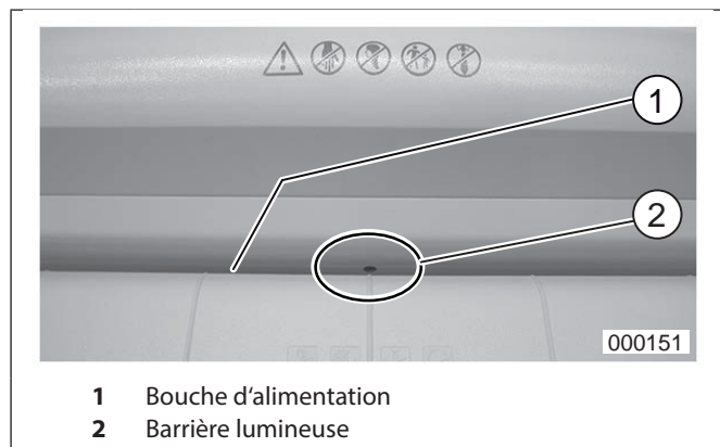
fig.3 Barrière lumineuse
