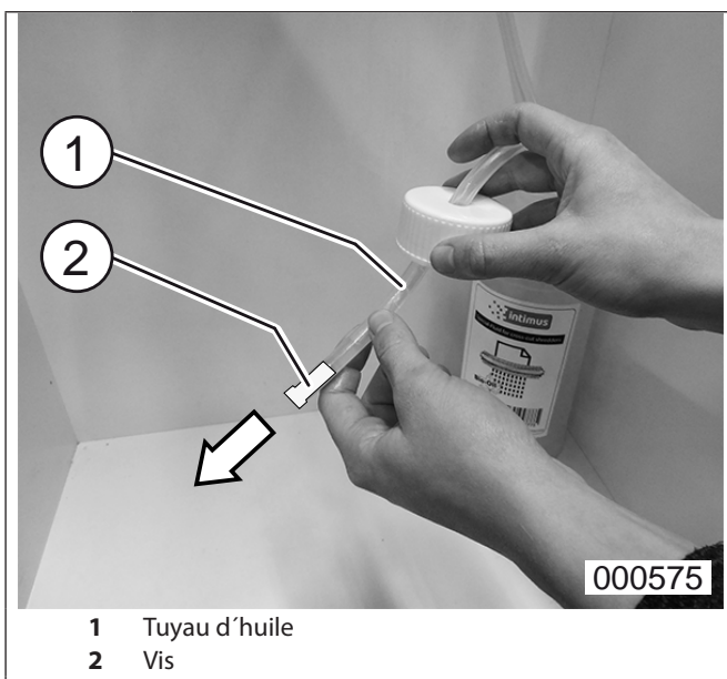
fig.1 Le montage du tuyau d'huile
