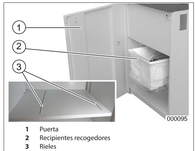
Fig. 4 Recipientes recogedores
