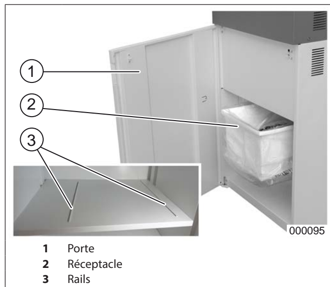
fig. 4 Réceptacle
